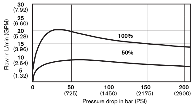
4WRAB6E12-1X
