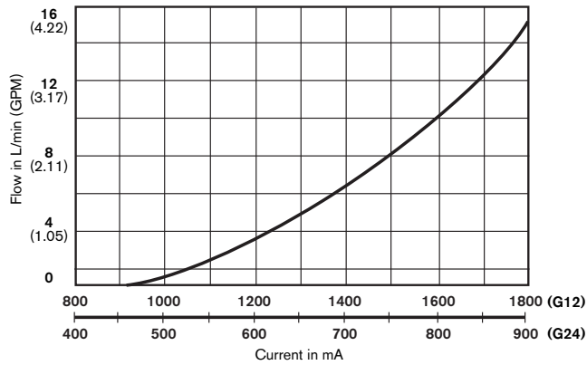
4WRAB6E12-1X
